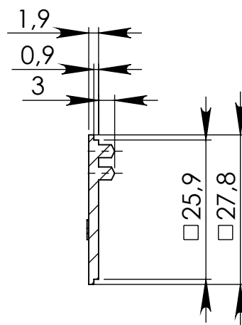
PRZEKRÓJ B-B
