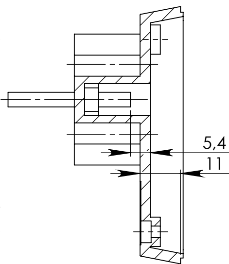
PRZEKRÓJ B-B SKALA 1 : 1
